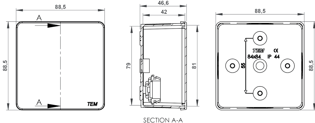
SECTION A-A
